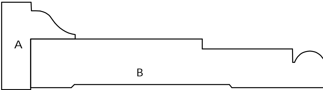
F-2863A,B A: 1.500" x 1.25" B: .8366" x 5.0145" O.A. 1.500" x 5.500" TW Perry
